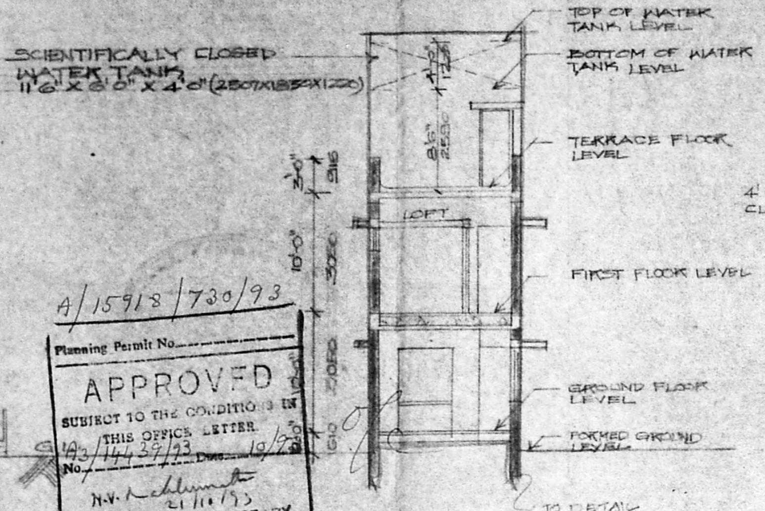
SECTION 'AB'
